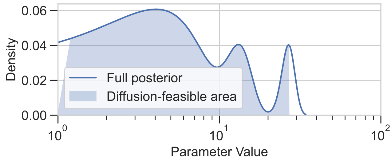
a2: Posterior with Diffusion-Feasible Area
